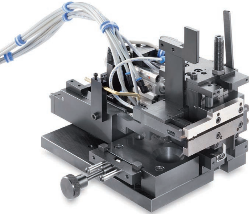
Abisoliermodul 517 mit Skalerrädern zur präzisen und schnellen Einstellung der Abisolierparameter
