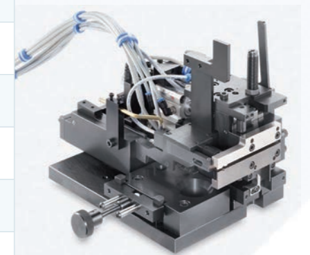
Abisoliermodul 517
