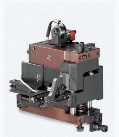
Abisoliermodul 512
